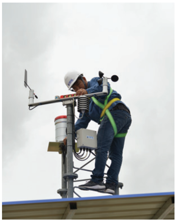
เครื่องมือ Weather Station Installation
